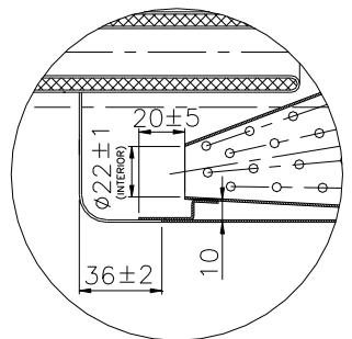
DETALLE A
